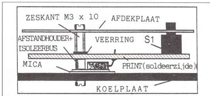
Figuur 3: Een doorsnede.
